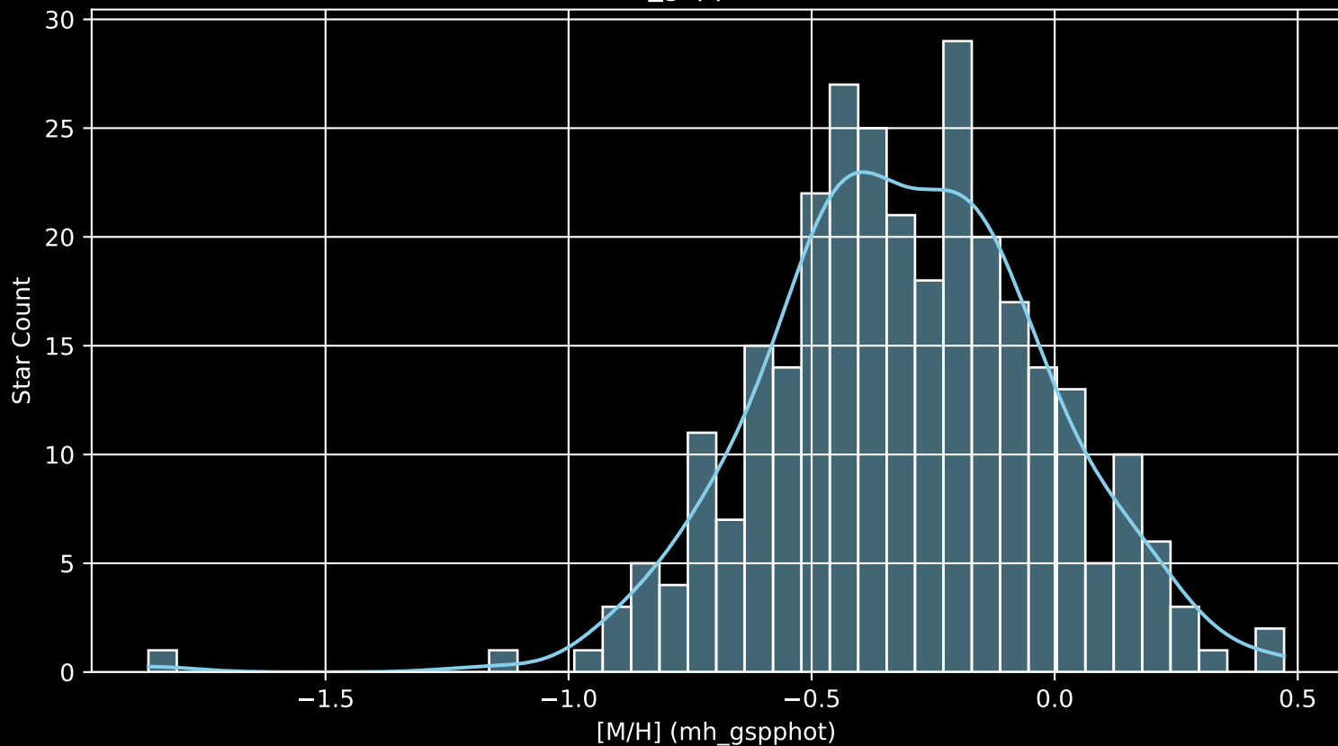
GALAH DR4 Field: [133] [M/H] (mh_gspphot) (n= 295)
